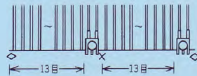
メリヤスカムの配置図
