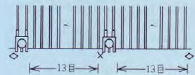
メリヤスカムの配置図
