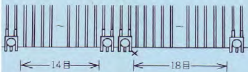
メリヤスカムの配置図
