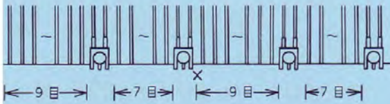
メリヤスカムの配置図
