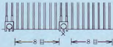
メリヤスカムの配置図
