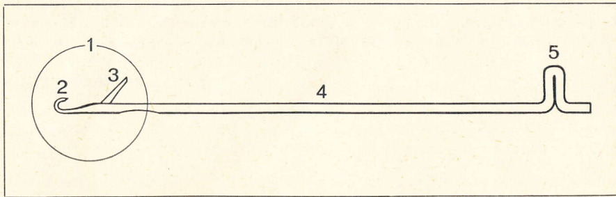
1 = Nadelkopf 2 = Häkchen 3 = bewegliche Zunge 4 = Nadelschaft 5 = Nadelfuss
