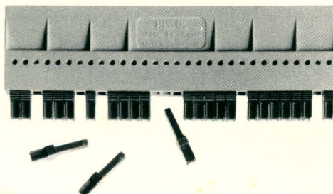
PASSAP WMK-61 Wechselmusterkamm Peigne sélecteur Pattern selector Regla selectora cambiabile
