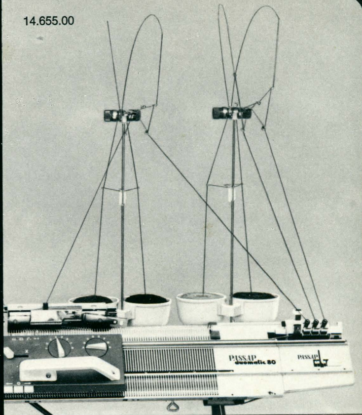
4-Farben-Wechsler Changeur automatique 4 couleurs Automatic 4-colour changer Cambiador automático de 4 colores
