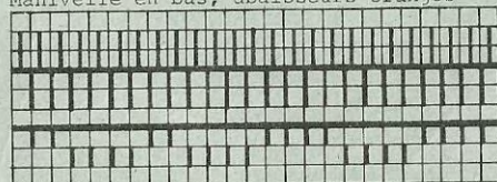
Schéma des mailles défaites Manivelle en bas, abaisseurs oranges
