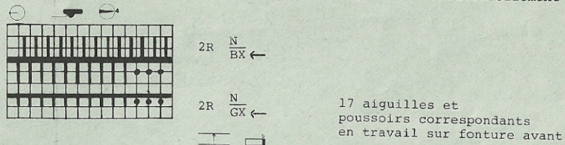
Schéma 2: Motif en relief avec carte Deco perforée individuellement
