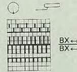
Schéma pour jacquard
