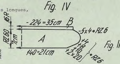
Schéma pour jacquard
