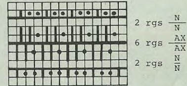
Schéma pour côte anglaise manivelle en haut, abaisseurs orange
