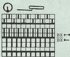
Schéma pour point jacquard uni (POINT 115)
