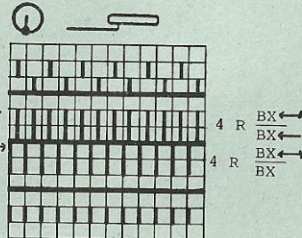
Schéma pour dessin 2 Jacquard uni (POINT 207)
